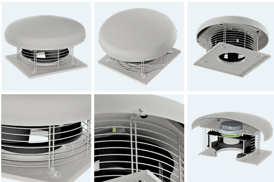
Siatka ochronna
